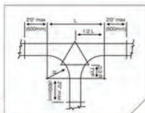
Horizontal Tee
